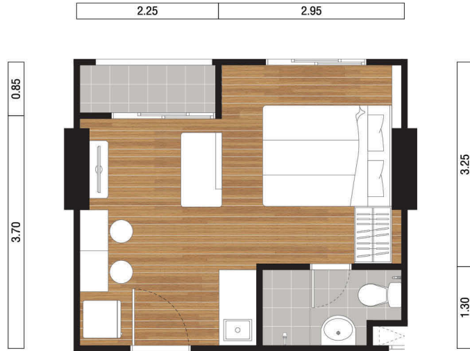
แบบห้องชุดขนาด 22.50 ตร.ม. ( อาคาร B )
