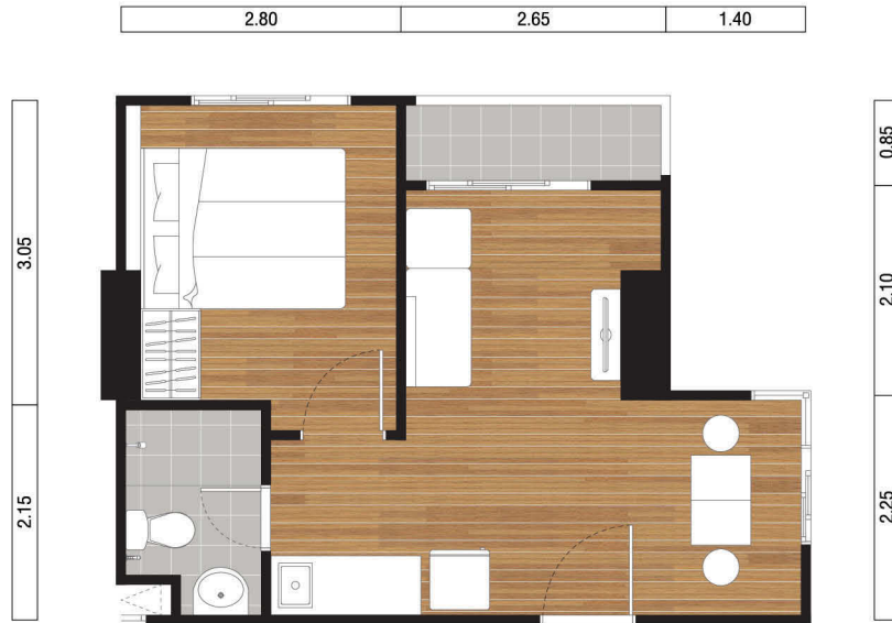
แบบห้องชุดขนาด 30.00 ตร.ม. ( อาคาร B )
